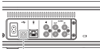
USB 포트
